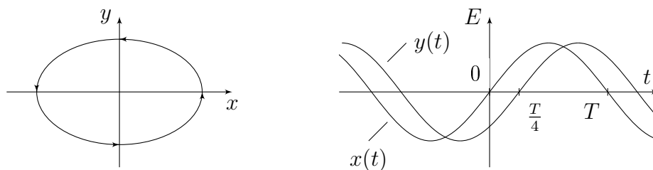
Рис. 10: Эллипс поляризации и графики компонент.
